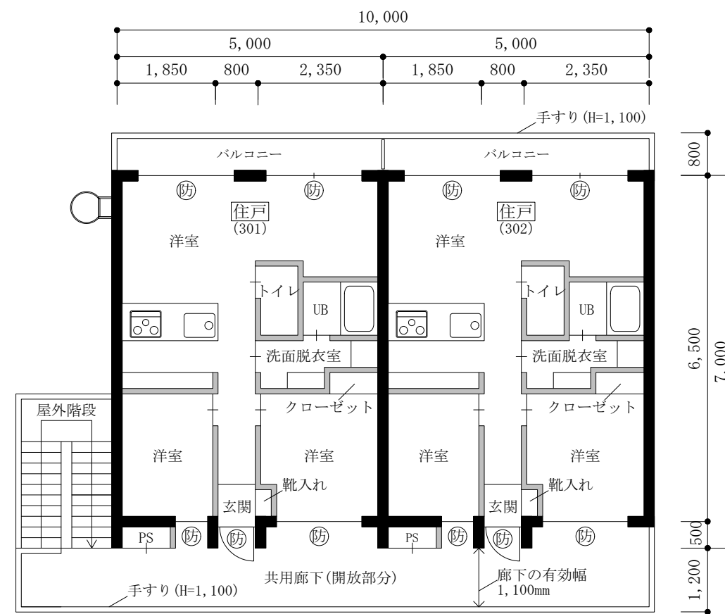
3階平面図
