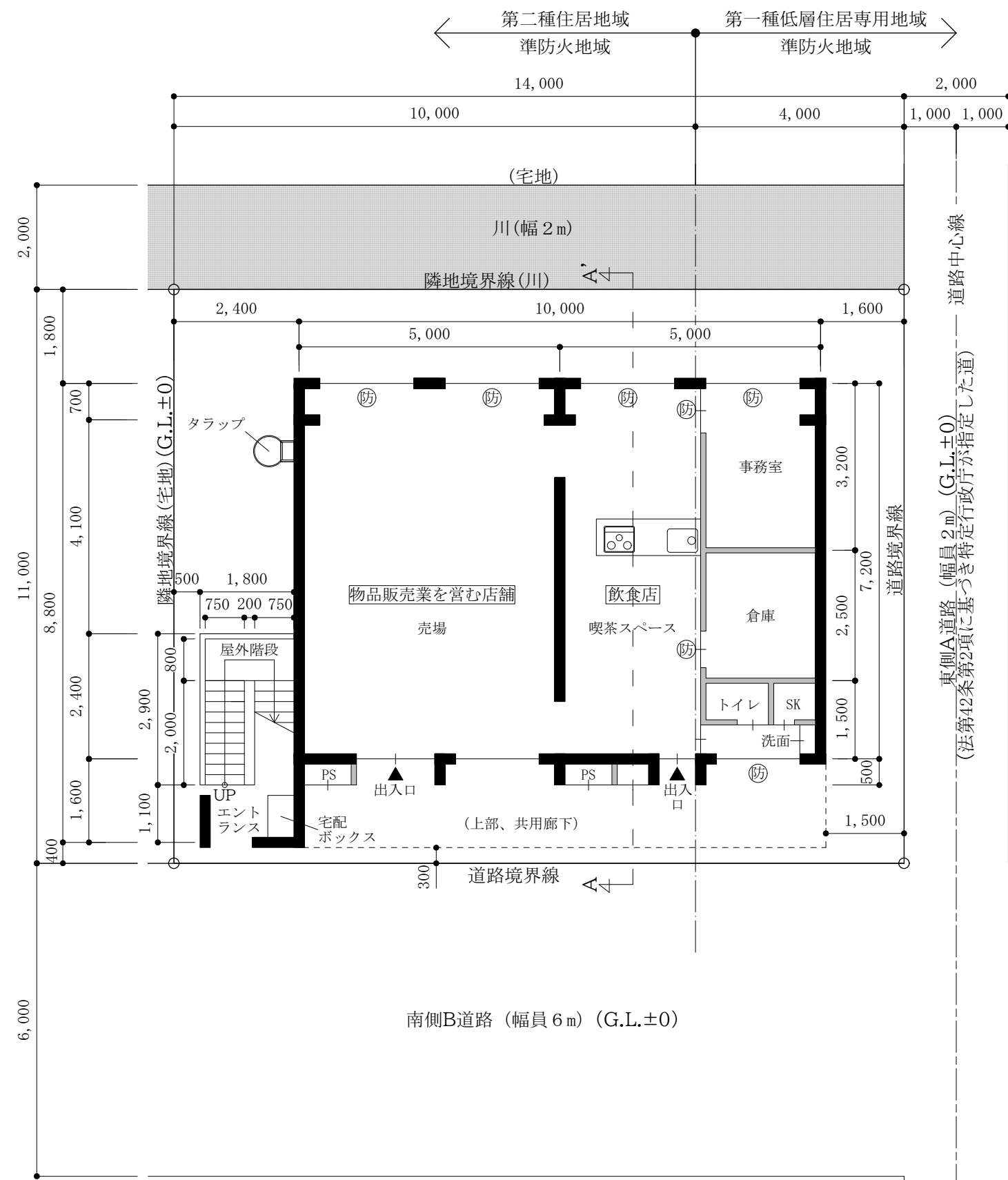
1階平面図・配置図
