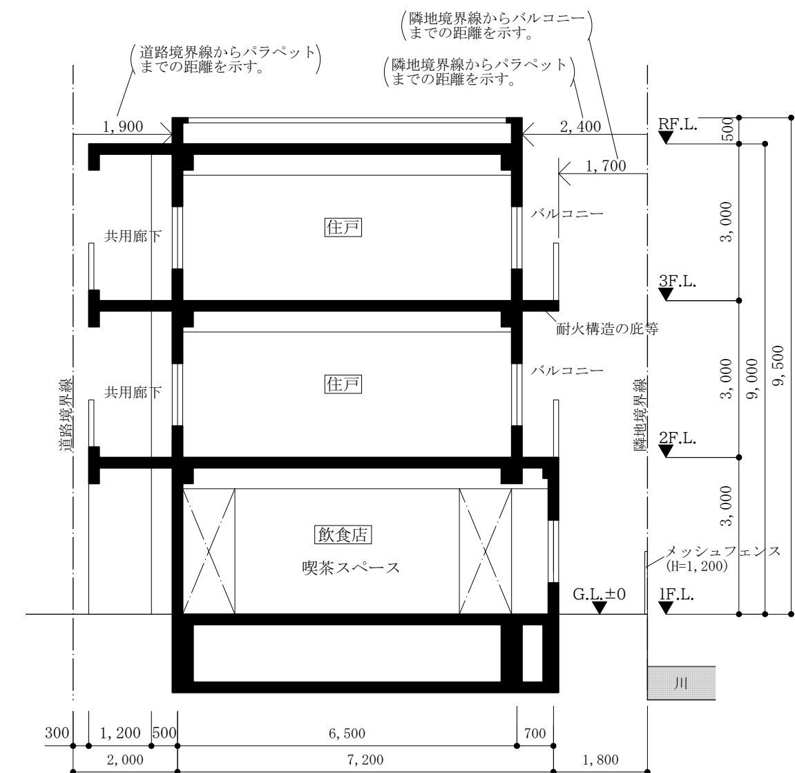
A-A'断面図
