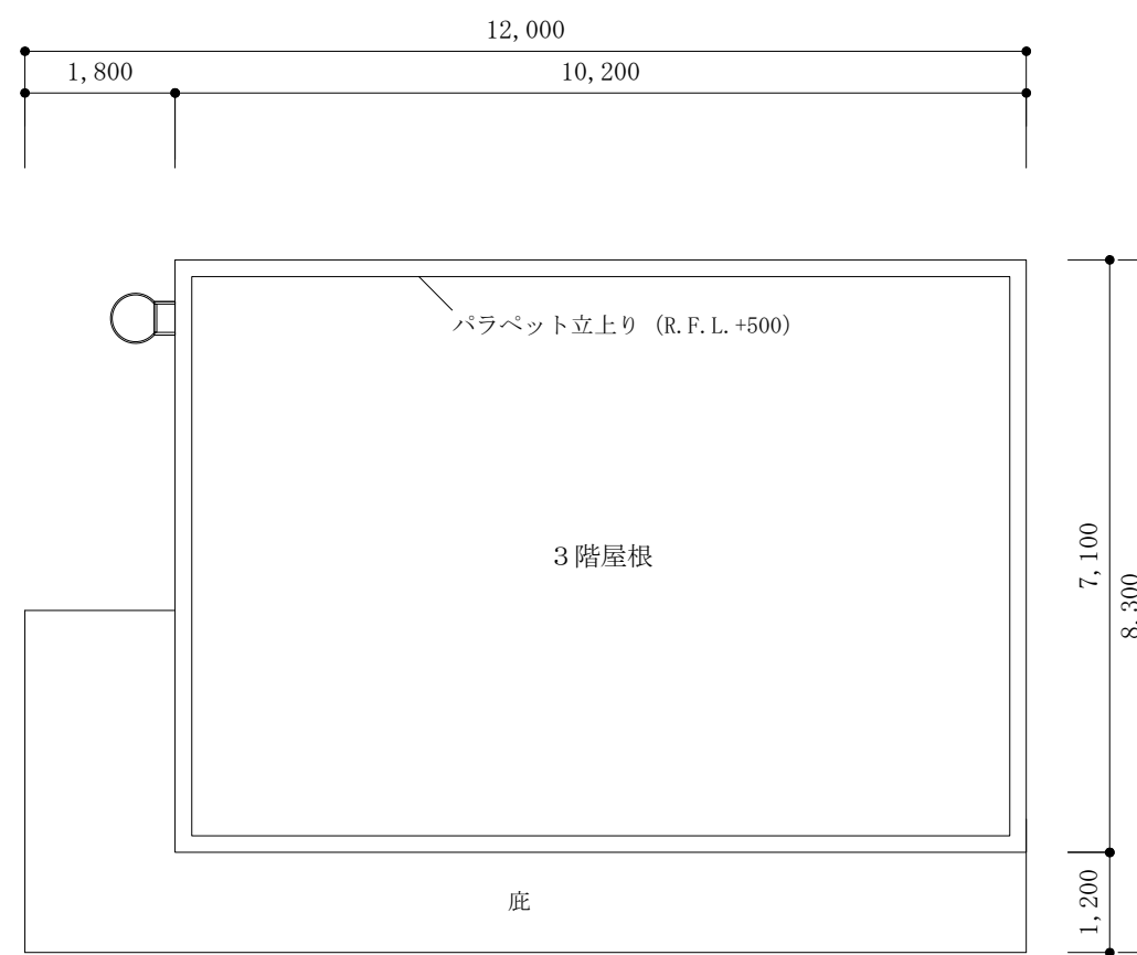
屋上階平面図
