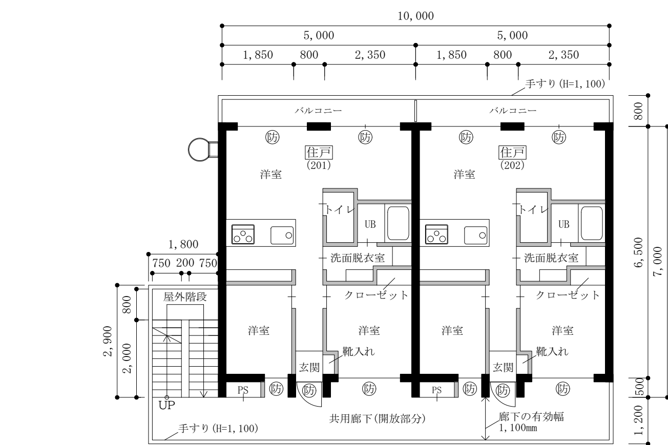
2階平面図
